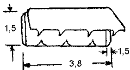
Προστατευτικό περίβλημα
